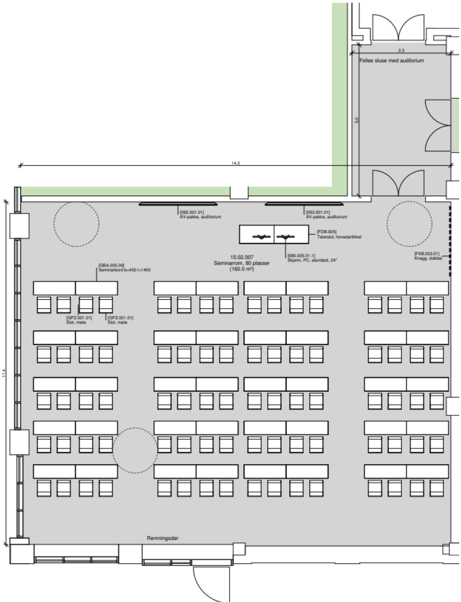
Planutsnitt 15.02.007 Seminarrom
