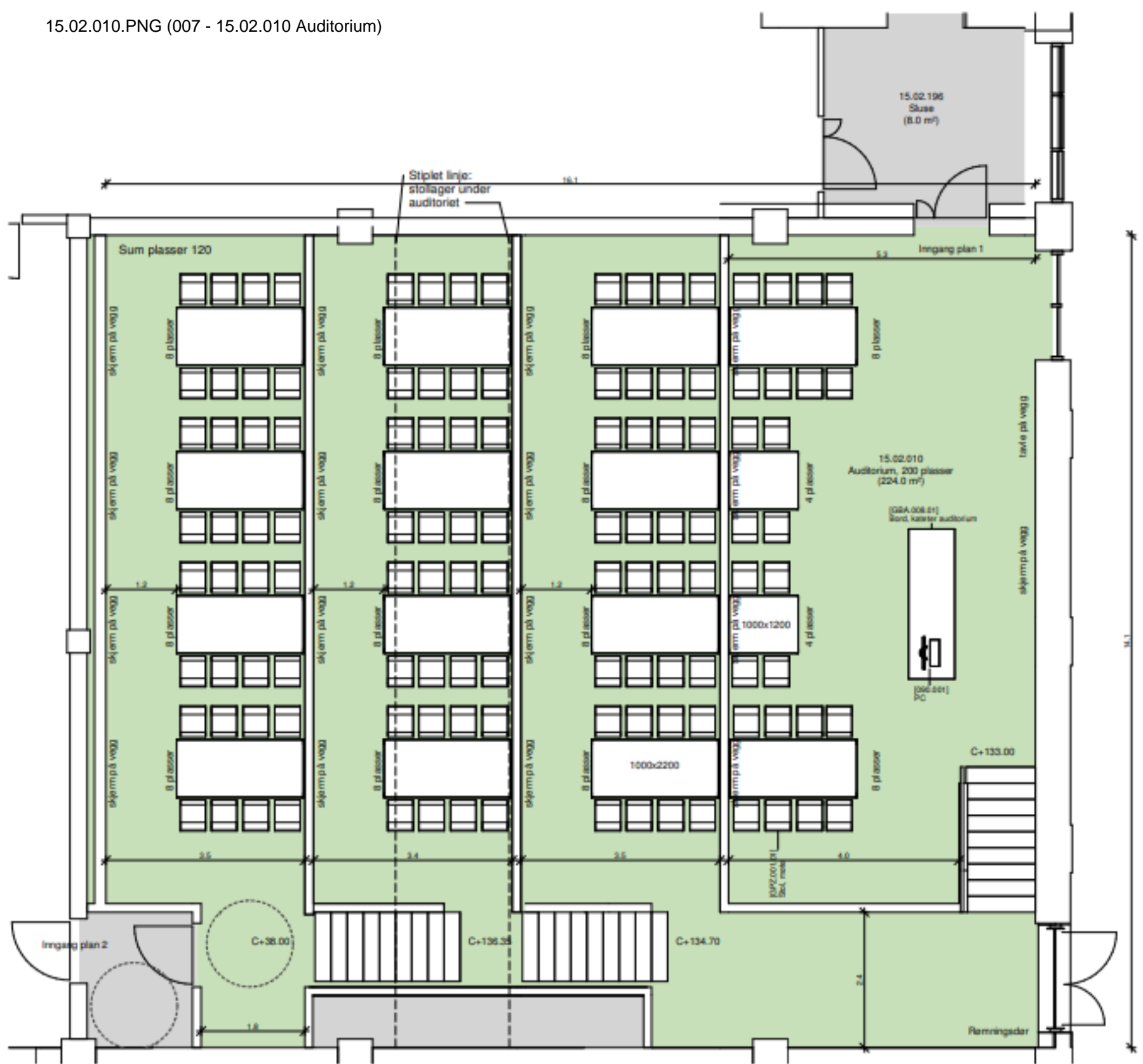
Planutsnitt 15.02.010 Auditorium 200 plasser
