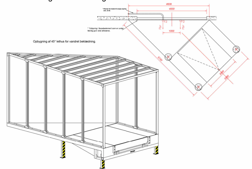
Porthus 6,7 og 8 stålunderstøttede/rampe. 45° Tette flaps utvendig og isolert leddport med varmluftsgardin innvendig.
