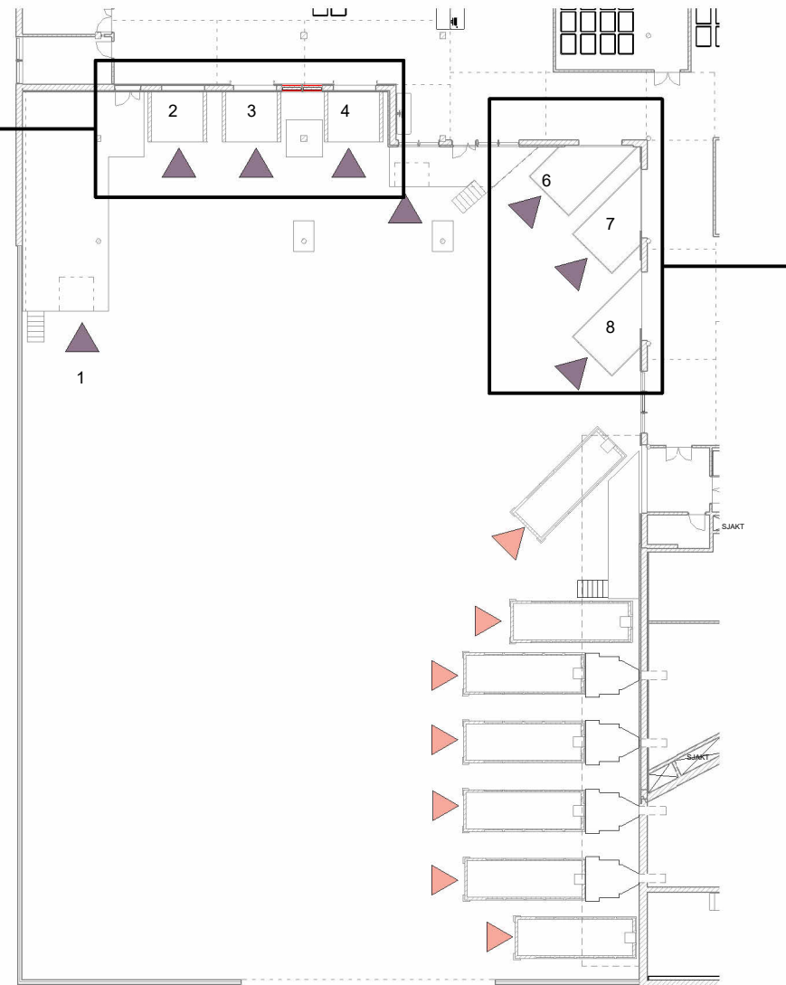
Porthus 6,7 og 8 stålunderstøttede/rampe. 45° Tette flaps utvendig og isolert leddport med varmluftsgardin innvendig.
