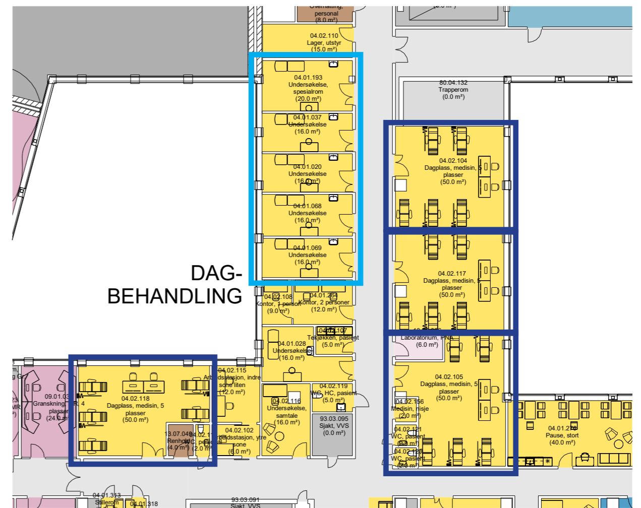
Plan 1 - nordøst
